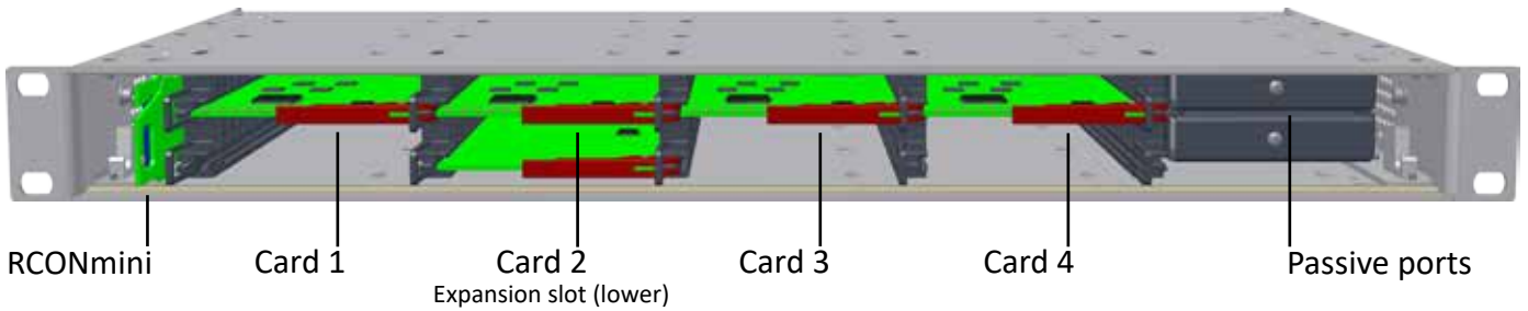
miniHUB-1RU-4-2
